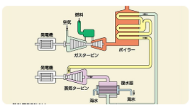
① GTCC発電
